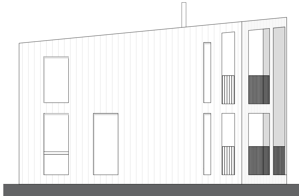
ELEVATION B
